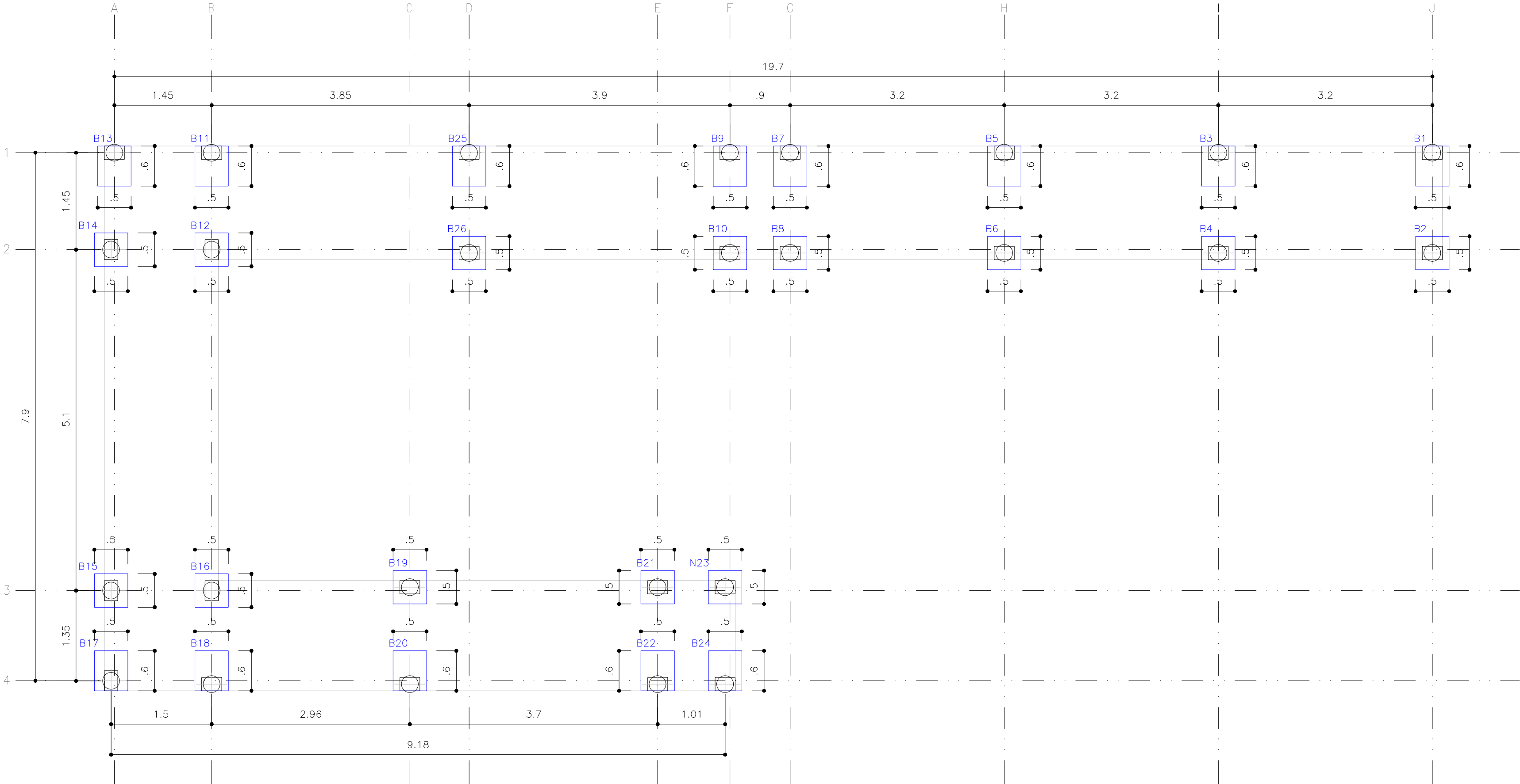
PLANTA DE LOCAÇÃO E DETALHAMENTO DOS BLOCOS DE COROAMENTO Esc 1:50
